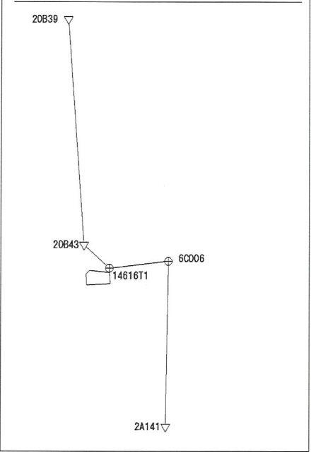
基準点網図 S=1/3000
